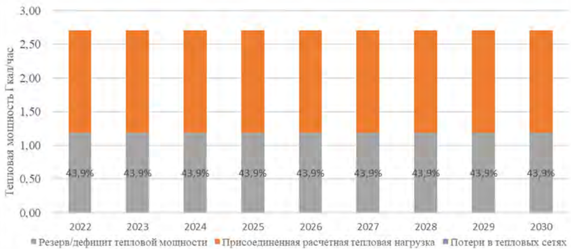
Рисунок 9 Баланс тепловой мощности и перспективной тепловой нагрузки котельной «Школьная»
