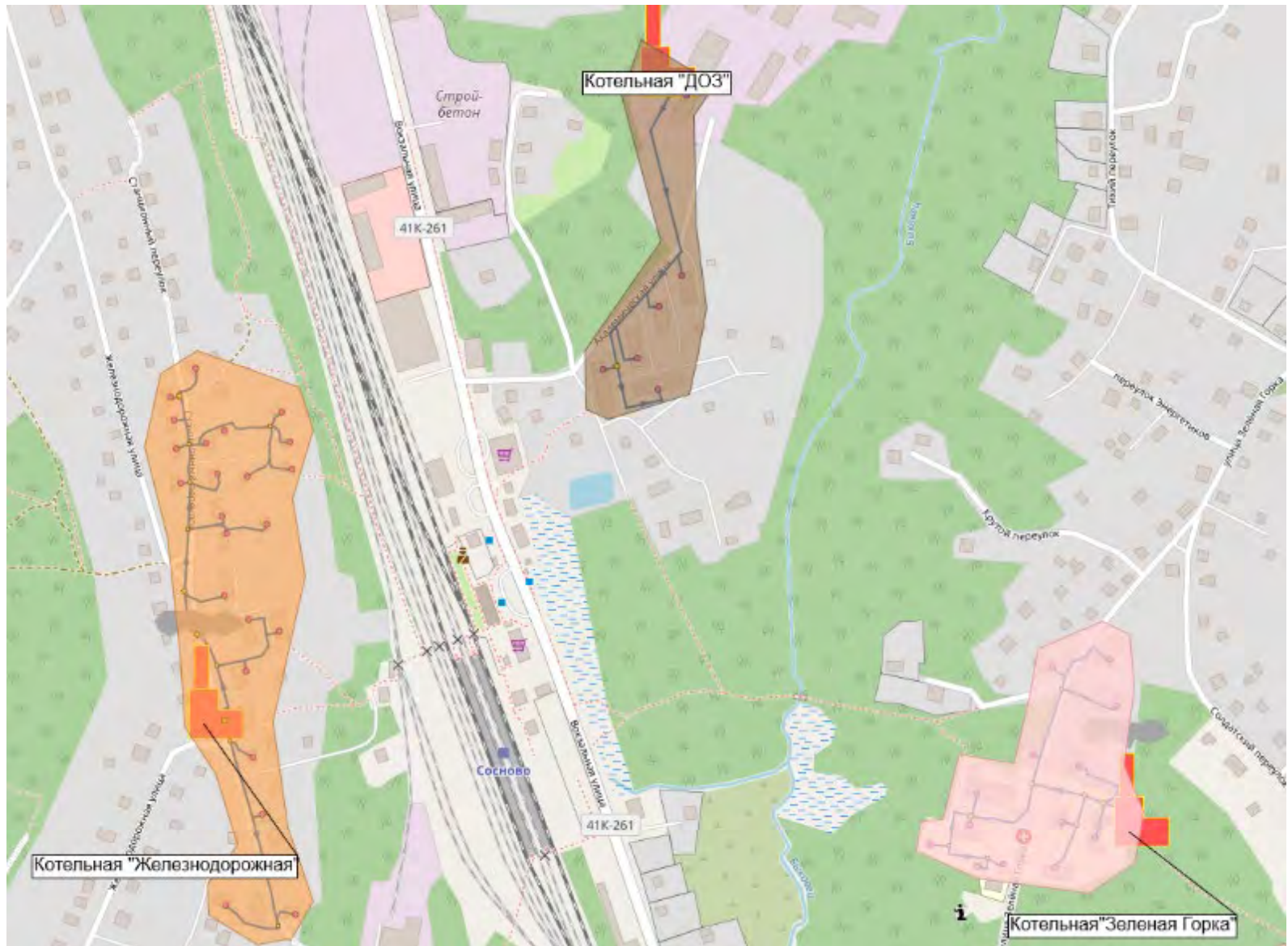
Рисунок 2 Зоны действия котельных «Железнодорожная», «ДОЗ», «Зеленая Горка»
