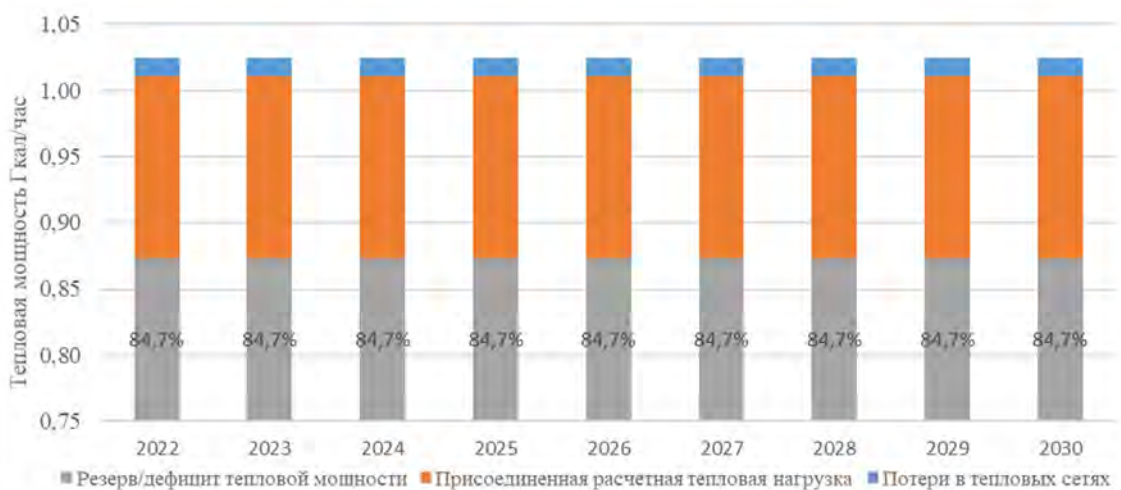
Рисунок 10 Баланс тепловой мощности и перспективной тепловой нагрузки котельной «Агрохим»
